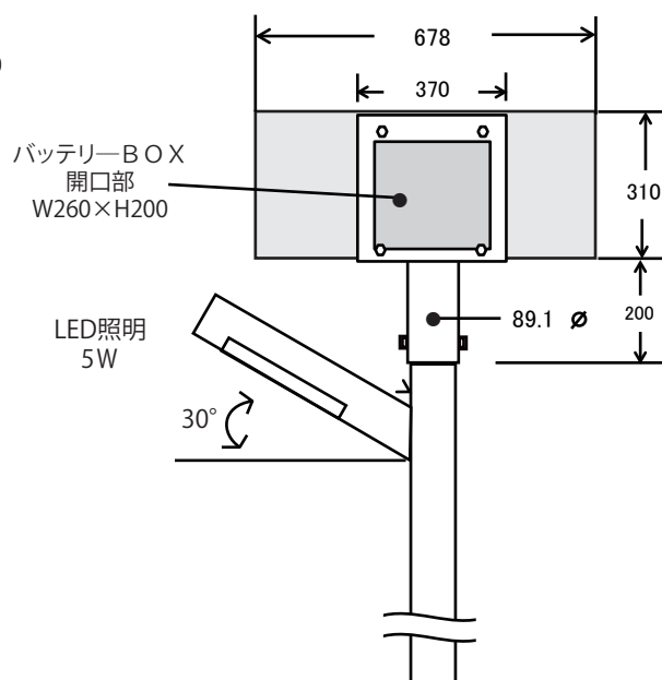
背面図
