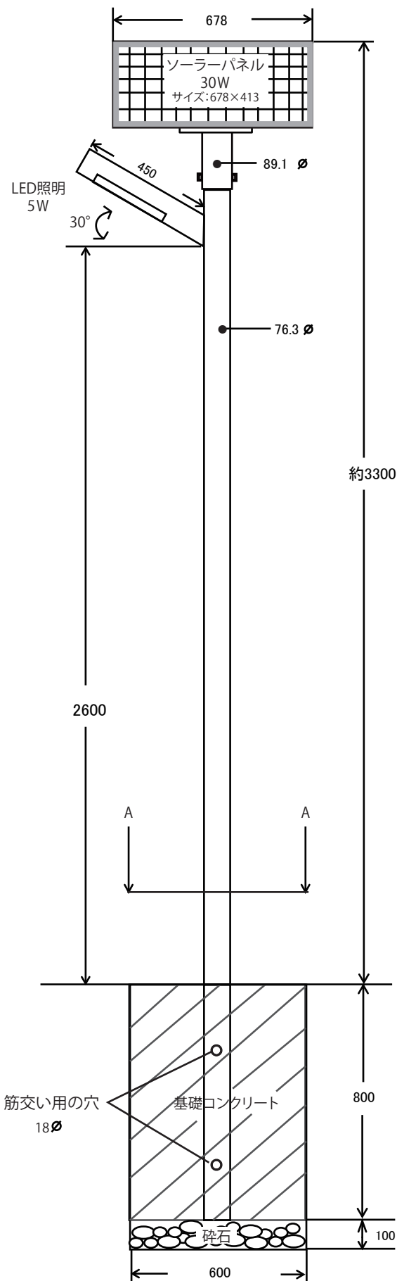
正面図
